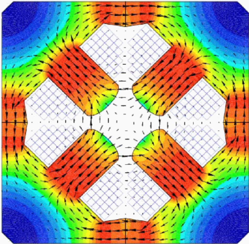
LEP quadrupole magnet (NC)
