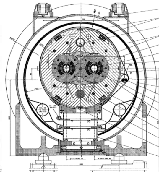
LHC
